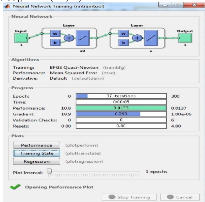
Рисунок 2 – Обучение сети
